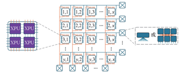
图 8 x \times y H \times 2 Mesh 网络 Fig. 8 x \times y H \times 2 Mesh network
