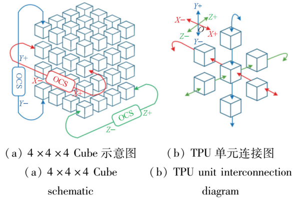
图9 谷歌 TPU Cube 和单元示意图
