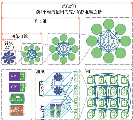
图 15 UB-Mesh 组示意图
