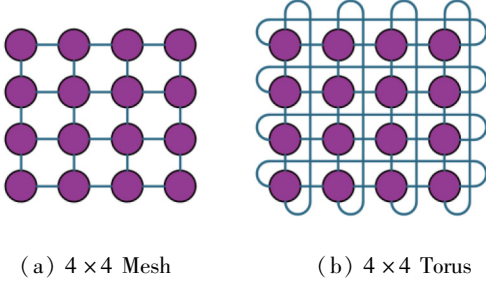
图4 4×4 Mesh 和 Torus 网络示意图 Fig. 4 Illustration of 4×4 Mesh and Torus networks
