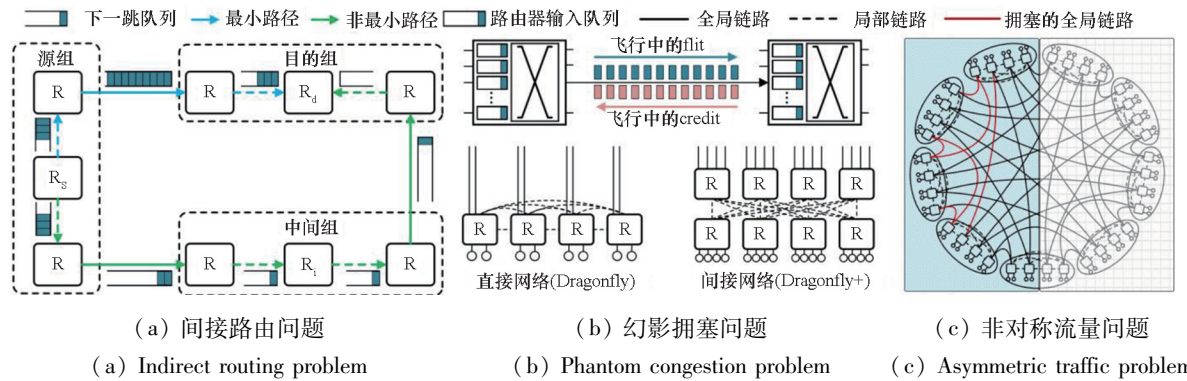
图 16 UGAL 在 Dragonfly 网络的三个问题
