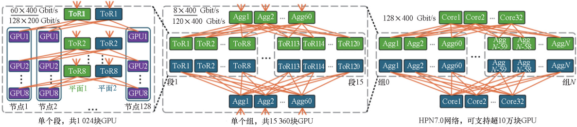
图 11 阿里巴巴 HPN7.0 网络 Fig. 11 Alibaba HPN7.0 network
