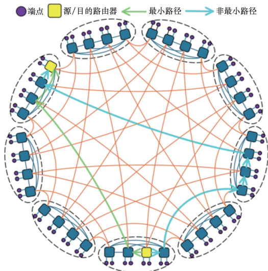
图 6 Dragonfly(4, 2, 2, 9)网络及其最小和非最小路径
