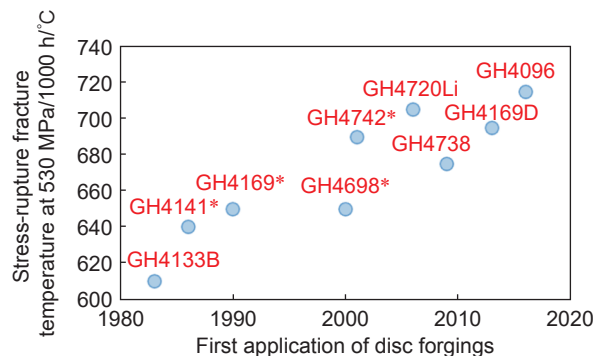
图 2 航空发动机及燃气轮机盘锻件用变形高温合金的发展趋势(*航天兼用) [21]
