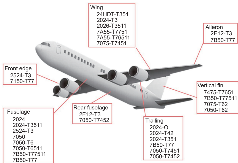
图3 航空主干铝合金在飞机上的应用部位
